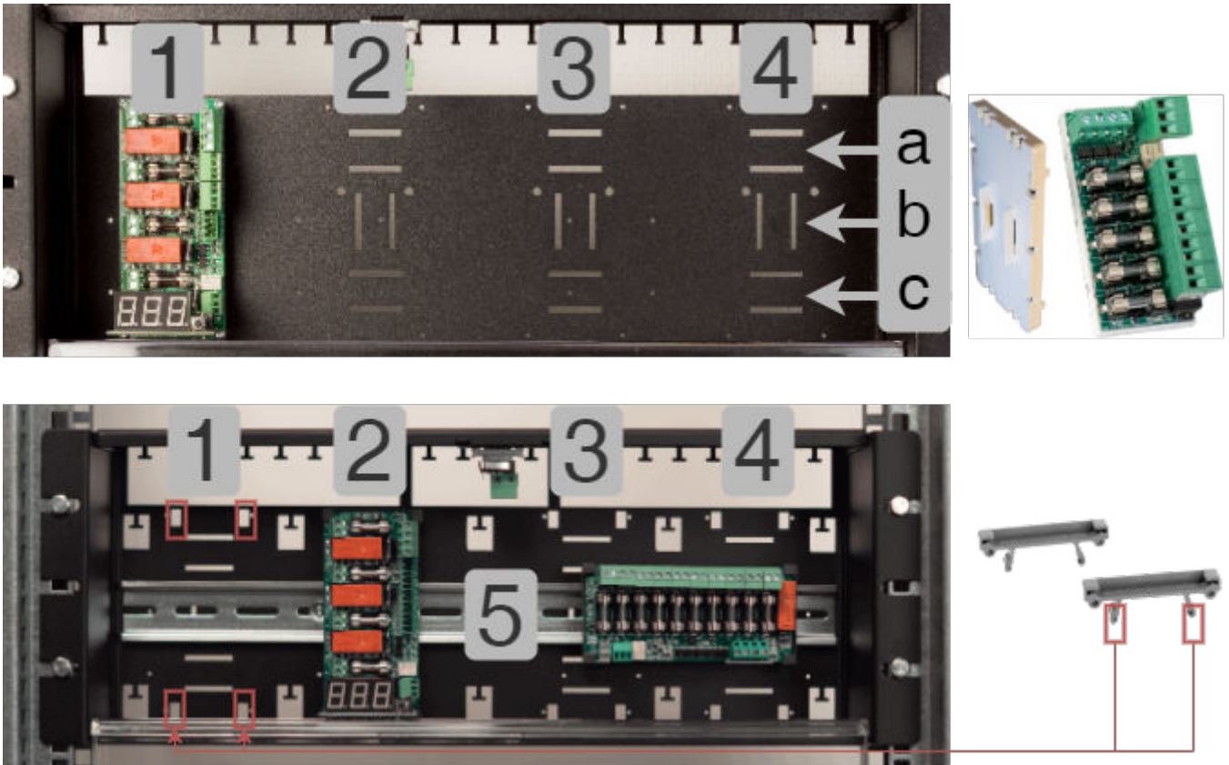
Figur 1. 19 rack module holder med diverse kort monteret.
